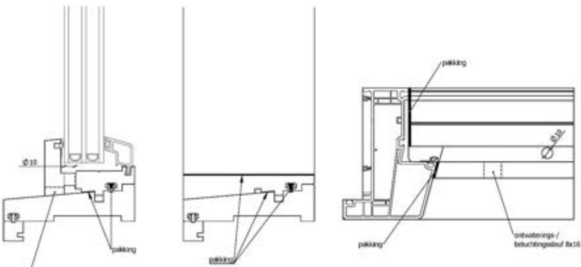
VAST GLAS
