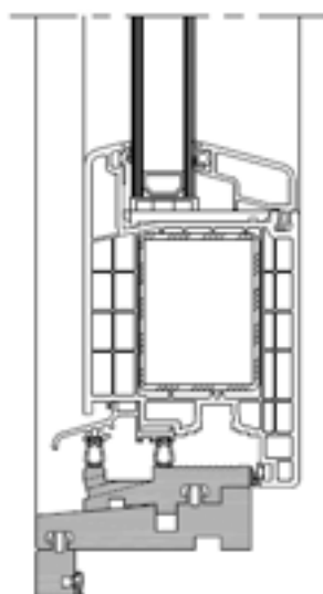
Binnendraaiende deur
