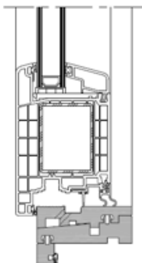
Buitendraaiende deur
