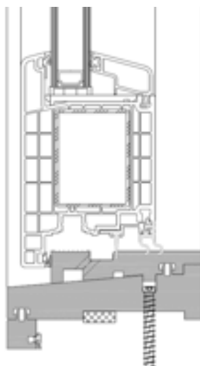
Buitendraaiende deur
