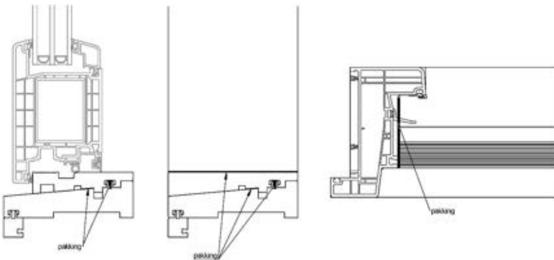
BUITENDRAAIENDE DEUR
