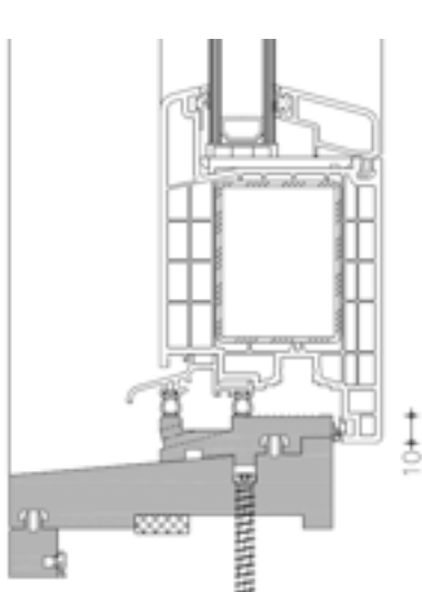
Binnendraaiende deur
